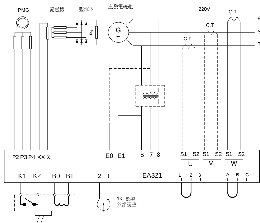
圖三 發電器接線圖
