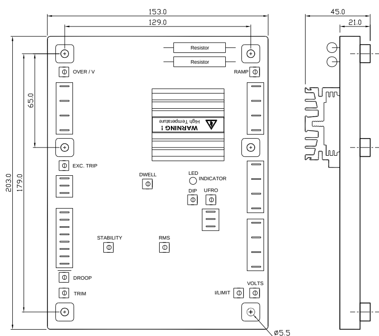
圖一 尺寸圖
